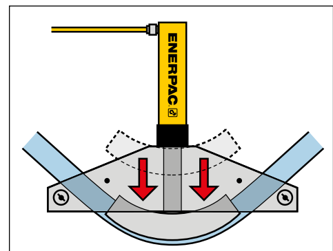
▲ Una tipica piegatura con sella a solo colpo.
